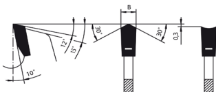
Zahnform
